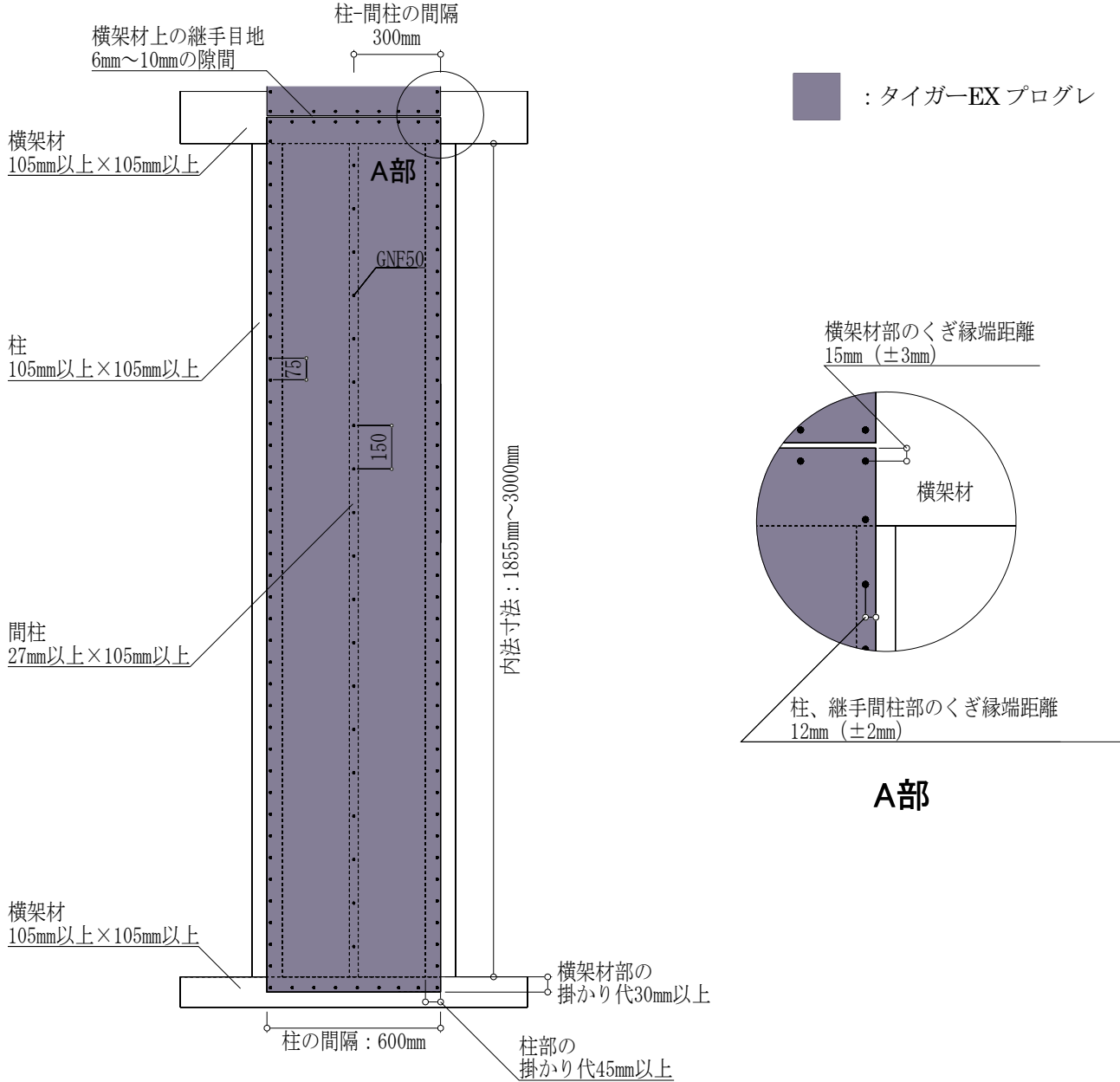
図6 標準仕様（FRM-0780：3.0倍） 施工概略図
